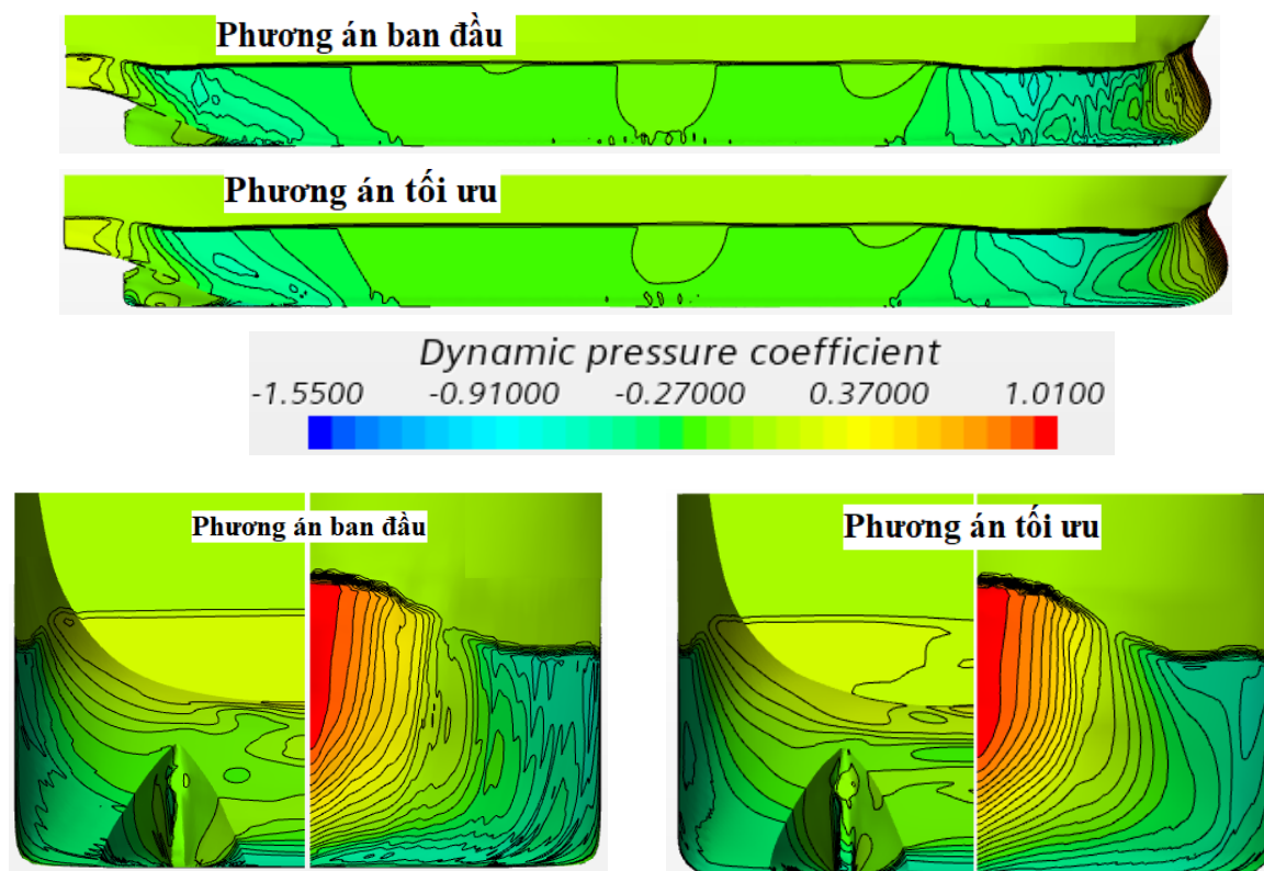
Hình 4.23. Sự khác nhau về phân bố C_P trên vỏ tàu giữa phương án ban đầu và phương án tối ưu khi tàu chạy trong luồng Cẩm Phả ở tốc độ 9,0 knots
