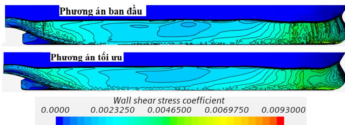
Hình 4.27. Sự khác nhau về phân bố C_F trên vỏ tàu giữa phương án ban đầu và phương án tối ưu khi tàu chạy trong luồng Cẩm Phả ở tốc độ 9,0 knots
