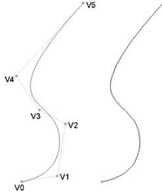
Hình 2.11. Điểm điều khiển được sử dụng trong việc tạo ra các phương án mũi quả lê
