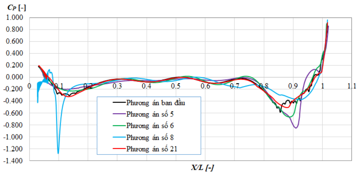
Hình 4.10. Phân bố áp suất thủy động trên bề mặt vỏ tàu ở các phương án khác nhau
