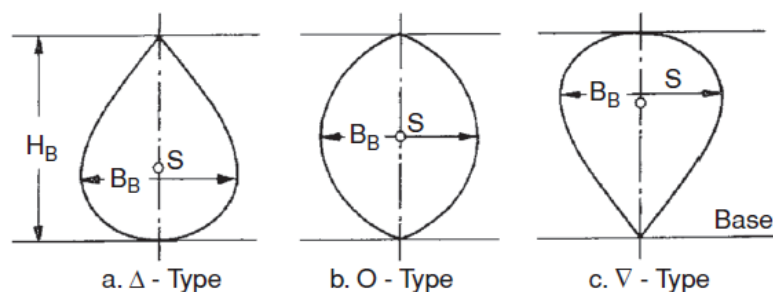
Hình 2.6. Hình dạng 3 loại mũi quả lê
