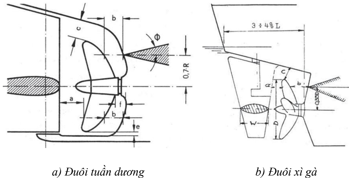
Hình 2.7. Các loại hình dáng đuôi tàu
