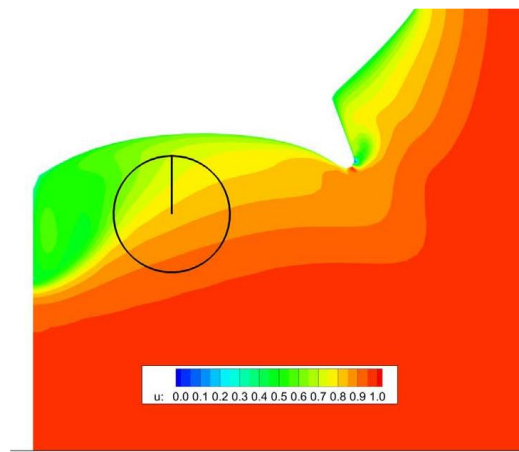
b) Hình dáng đáy chữ V, h/T=3,0
