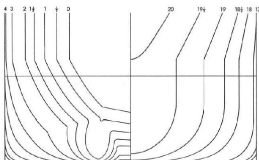
Hình 2.9. Phần đuôi thân tàu SSPA được thiết kế để sử dụng hai chong chóng [12]
