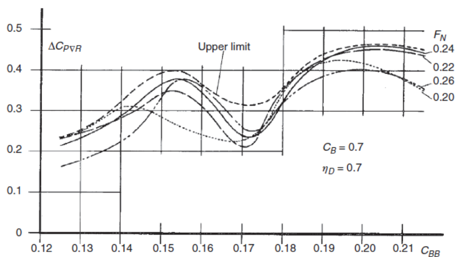
Hình 1.7. Ảnh hưởng của tham số C_{BB} mũi quả lê đến \Delta C_{PVR} của tàu
