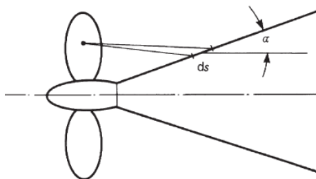
Hình 2.8. Ảnh hưởng của lực hút chong chóng lên thân tàu
