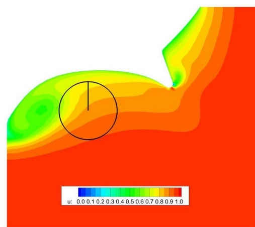
a) Hình dáng đáy chữ S, h/T=3,0
