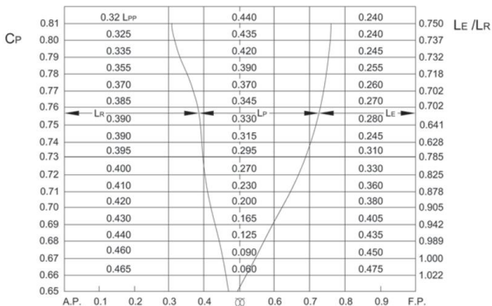
Hình 1.4. Khuyến nghị lựa chọn chiều dài đoạn thân ống, chiều dài phía mũi và đuôi tàu với C_P khác nhau (áp dụng với tàu có L/B=7,0 )
