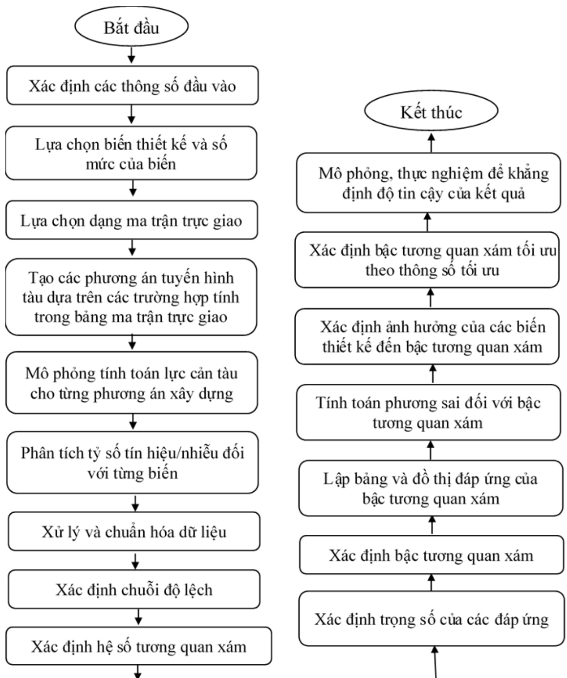
Hình 3.1. Quy trình các bước cải tiến hình dáng thân tàu hàng cấp VR-SB
