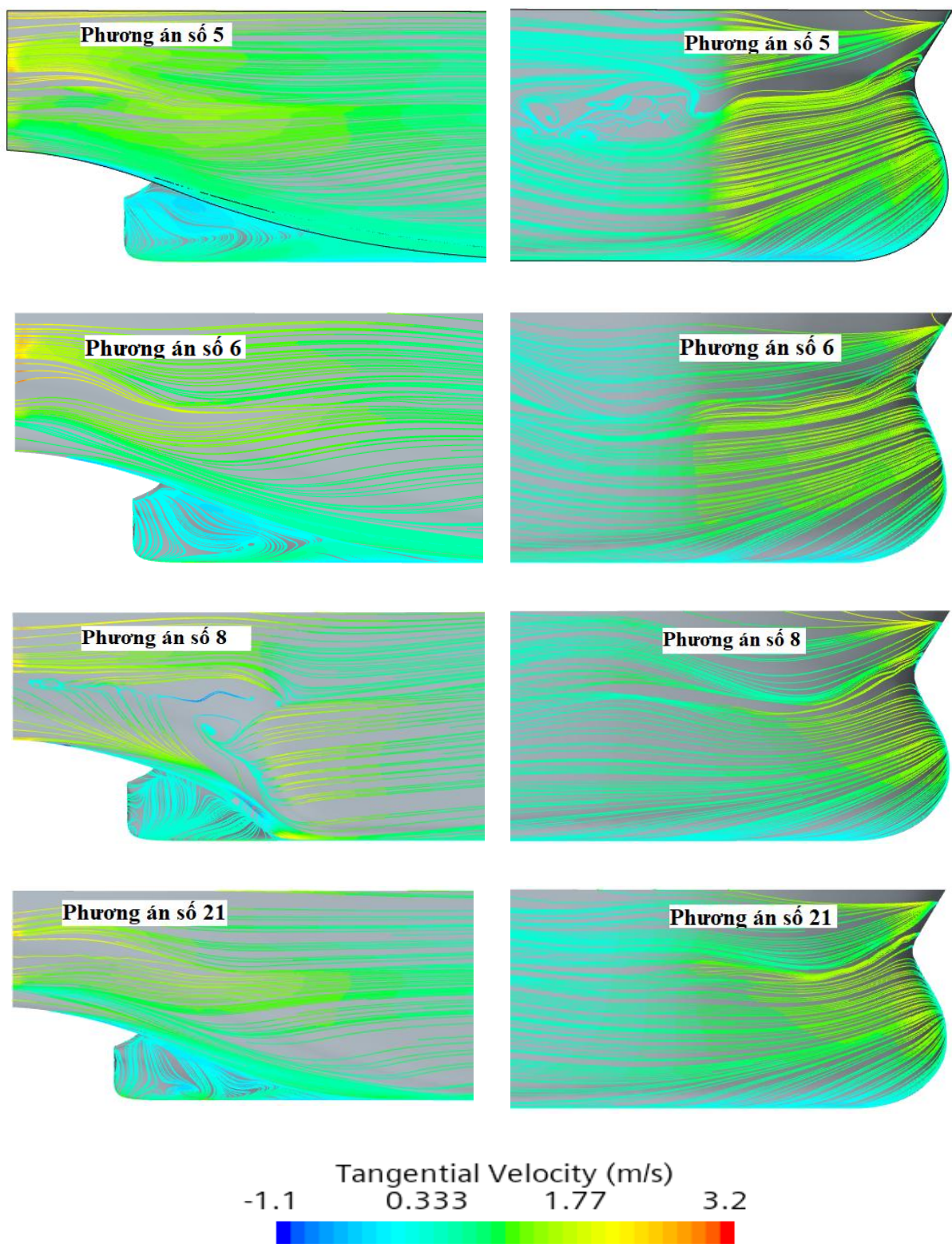
Hình 4.9. Đường dòng tại khu vực mũi và đuôi tàu khi chạy trong kênh Cẩm Phả
