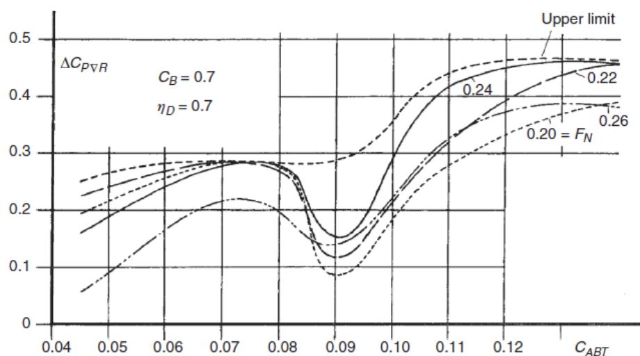
Hình 1.8. Ảnh hưởng của tham số C_{ABT} mũi quả lê đến \Delta C_{PVR} của tàu
