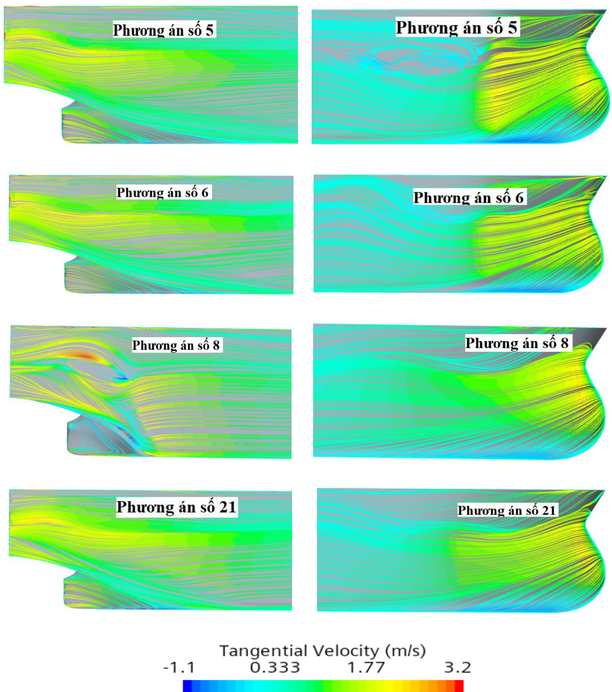
Hình 4.8. Đường dòng tại khu vực mũi và đuôi tàu khi chạy ngoài biển
