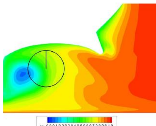
b) Hình dáng đáy chữ V, h/T=1,2
