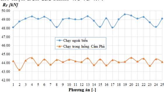
Hình 4.5. Kết quả mô phỏng tính toán thành phần lực cản ma sát tàu 4600 tấn ở các phương án khác nhau
